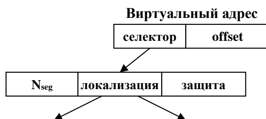
Рис. 142. Сегментно-страничное распределение. Упрощенная модель Intel.
