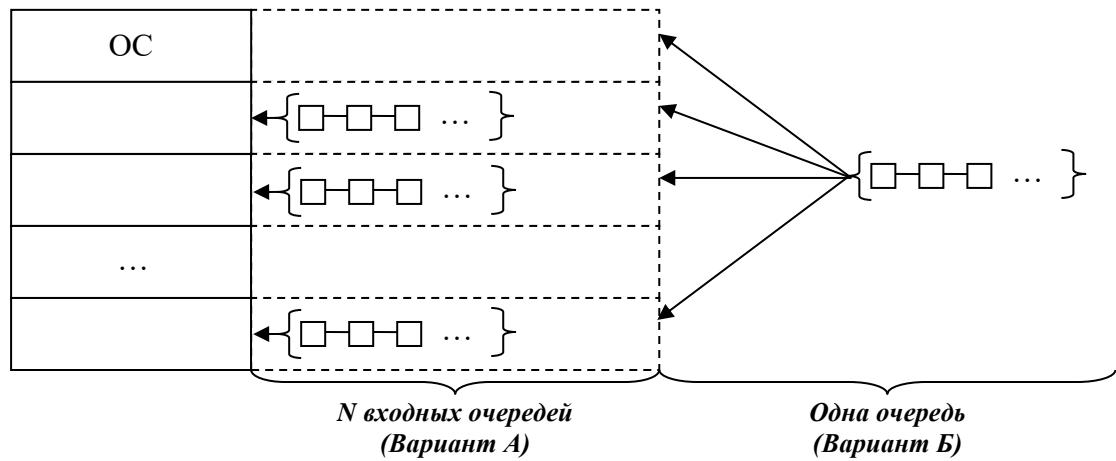
Рис. 132. Распределение неподвижными разделами.
