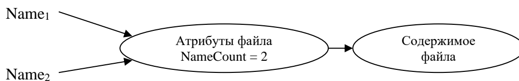
Рис. 111. Пример жесткой связи.
