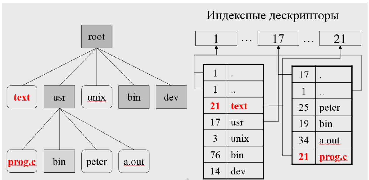
Рис. 124. Файл-каталог.
