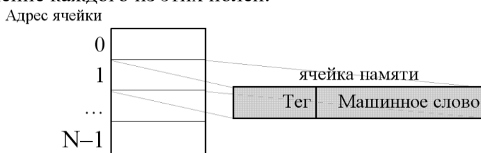
Рис. 22. Ячейка памяти.
