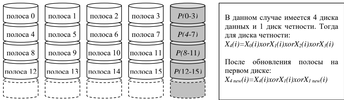
Рис. 155. RAID 4.
