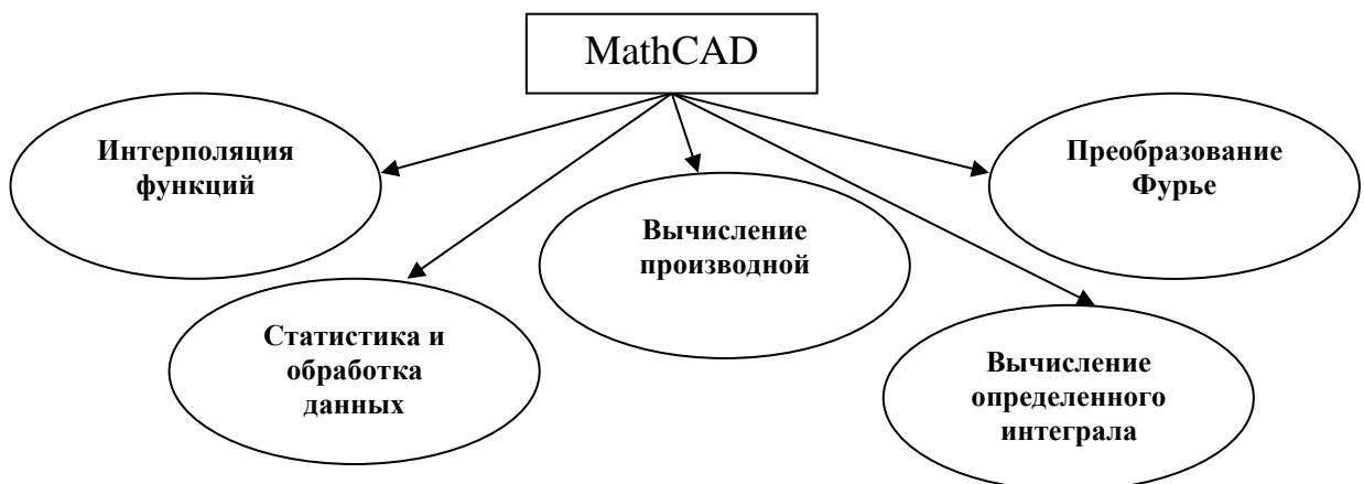
Рис. 17. Пакет MathCAD.
