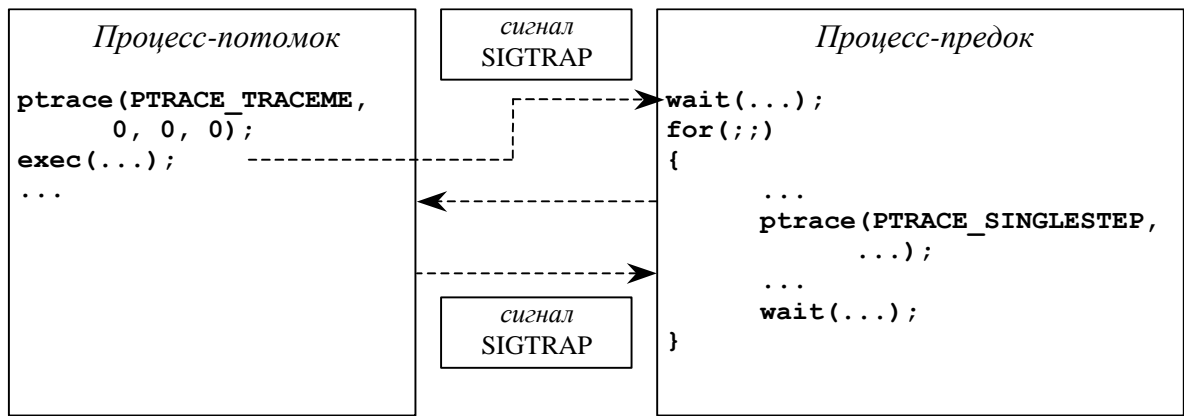
Рис. 98. Общая схема трассировки процессов.
