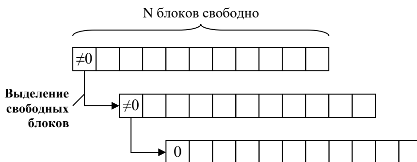
Рис. 121. Работа с массивами номеров свободных блоков.
