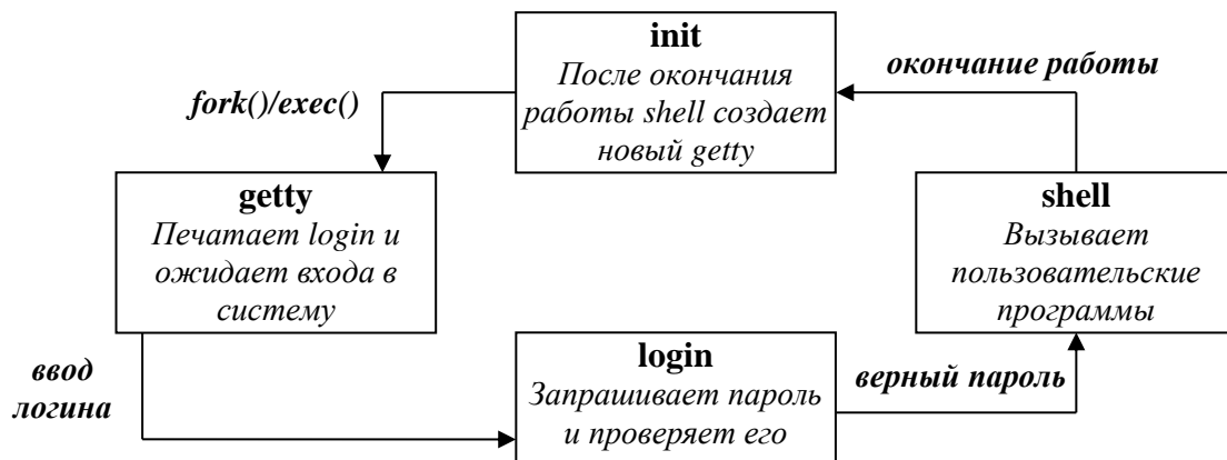
Рис. 90. Схема работы пользователя с ОС Unix.
