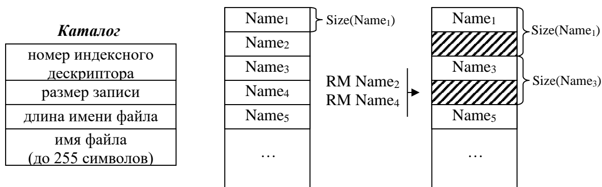
Рис. 130. Структура каталога FFS BSD.
