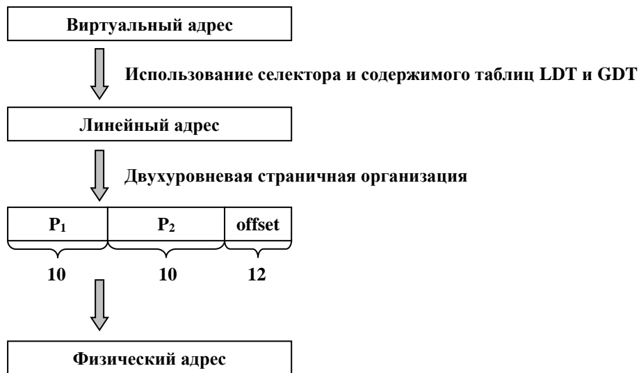
Рис. 143. Схема преобразования адресов.
