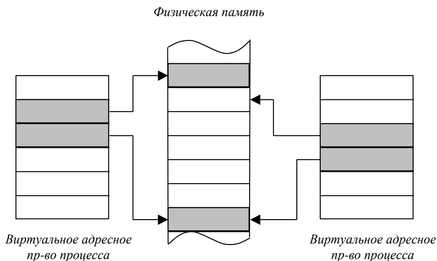
Рис. 100. Разделяемая память.
