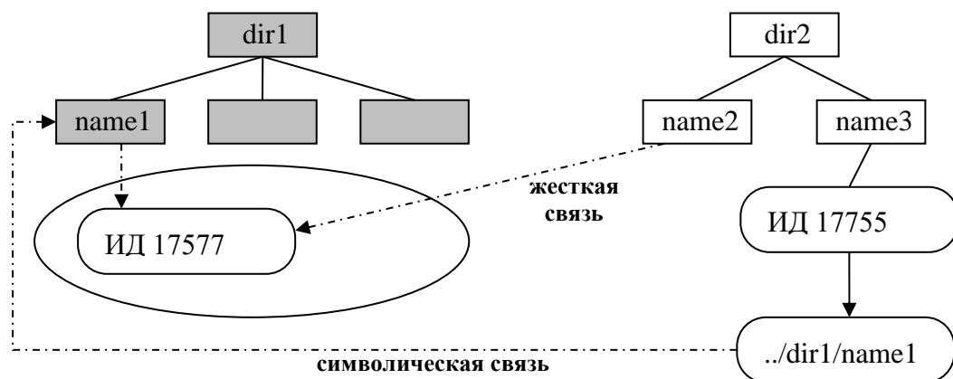
Рис. 125. Установление связей.
