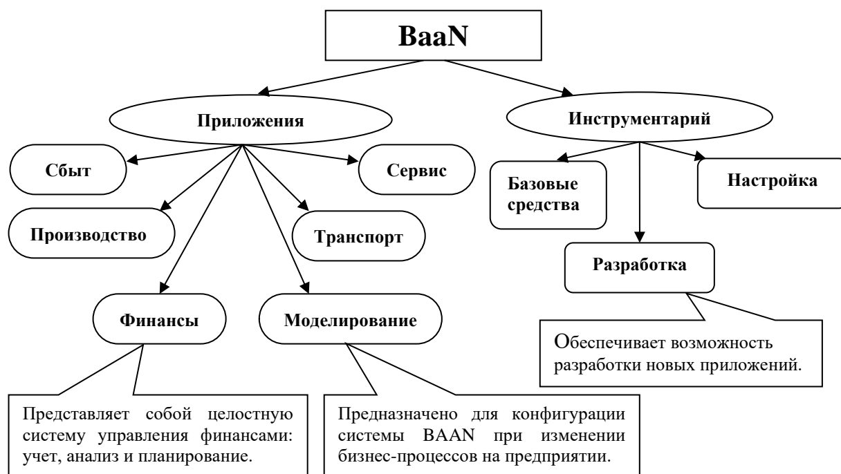
Рис. 18. Система ВааN.
